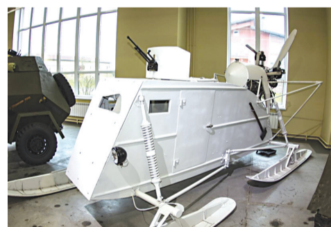
Боевые аэросани НКЛ-26, 1941 г.
